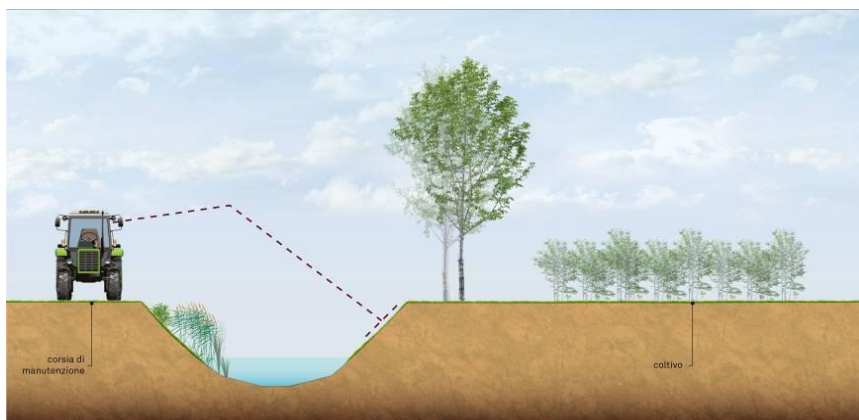
Figura 4 – Fascia arboreo-arbustiva posta sul ciglio di sponda su un solo lato di un canale o un capofosso; la manutenzione dell'alveo è eseguita dalla sponda opposta se la larghezza del canale lo consente, mentre quella della fascia boscata è operata dalla carreggiata presente sullo stesso lato della siepe (Immagine: Veneto Agricoltura).
