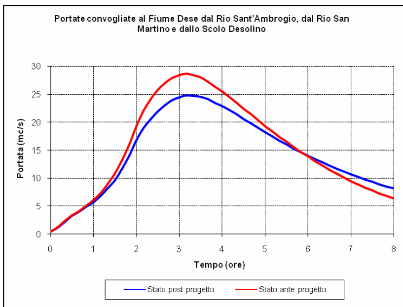
Figura 4 - Simulazione della riduzione dei picchi di piena convogliati al Fiume Dese dai tre affluenti interessati dagli interventi.
