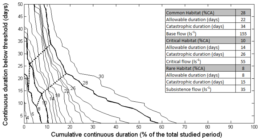
Figura 2 – Applicazione delle curve UCUT per il rio Valleritta (Roccasparvera, Cuneo) con riferimento al periodo di magra invernale (periodo simulato: 1 Gennaio - 21 Marzo tra il 1970 e il 2010, Vezza et al. , 2012c). Le rispettive soglie di valori di habitat disponibile per condizioni comuni (28%), critiche (10%) e catastrofiche (8%) sono espresse in termini di superficie bagnata dell'alveo inciso (CA%). La riduzione della pendenza nonché un aumento della spaziatura tra le curve indicano un aumento della frequenza di accadimento dell'evento sotto-soglia (Parasiewicz, 2007b) ed i punti di flesso delle curve selezionate vengono usati per definire le durate massime ammissibili (espresse in gorni, dettagli in, Parasiewicz, 2007b).
