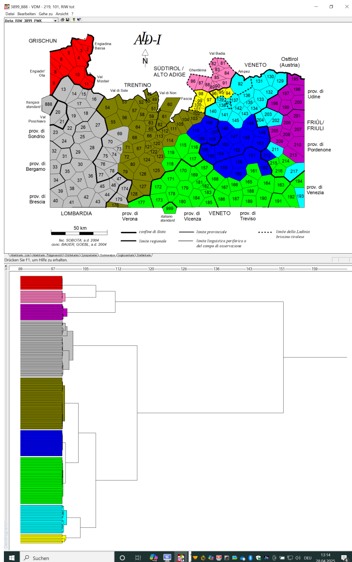
Karte 10 – Dendrographische Analyse nach der Methode von Joe Ward Jr. Beta-Dialektometrie: Ähnlichkeitsmessung: RIW + PMK (Produkt-Moment-Korrelations-Koeffizient [nach Bravais-Pearson]) Visualisierung: durch neun in Baum und Karte (analog zu Karte 9) ident eingefärbte Dendreme bzw. Choreme Korpus: 3.899 Arbeitskarten aus ALD-I (alle linguistischen Kategorien).
