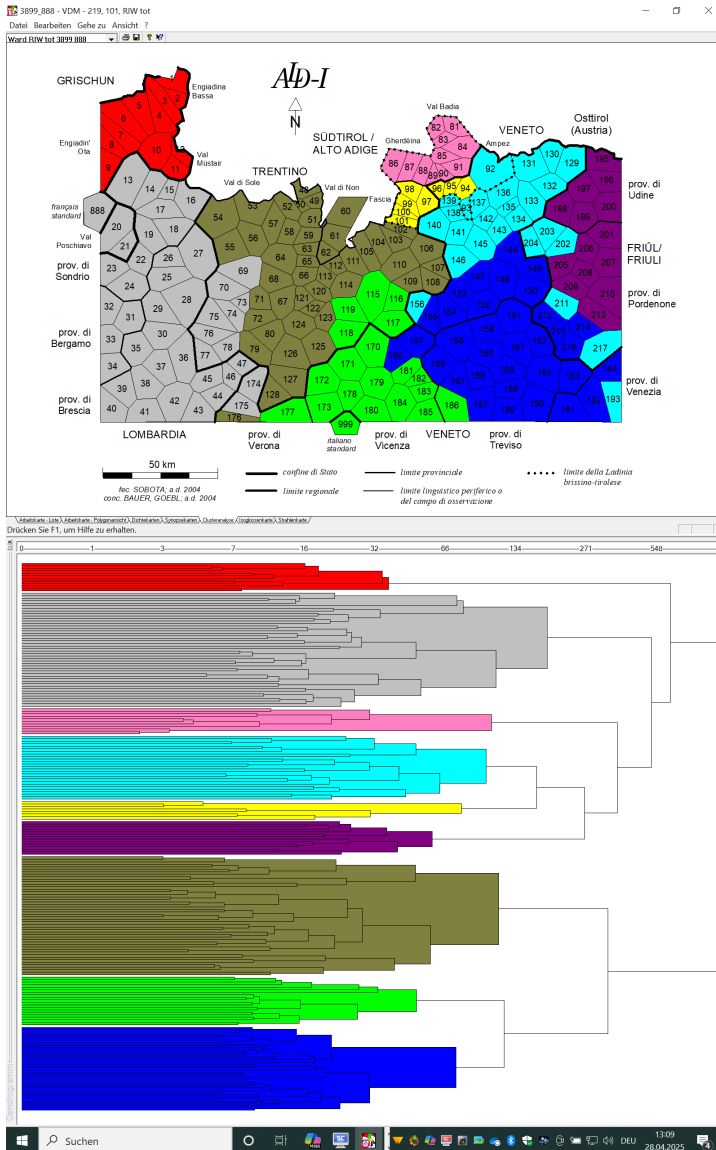
Karte 9 – Dendrographische Analyse nach der Methode von Joe Ward Jr. Alpha -Dialektometrie: Ähnlichkeitsmessung: R/W (Relativer Identitätswert) Visualisierung: durch neun in Baum und Karte (analog zu Karte10) ident eingefärbte Dendreme bzw. Choreme Korpus: 3.899 Arbeitskarten aus ALD-I (alle linguistischen Kategorien).
