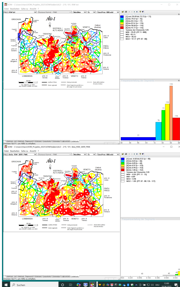
Karte 8 – Zwei Strahlen-Karten zum ALD-I: Messung der interpunktuellen Ähnlichkeiten Oben (Alpha-Dialektometrie): Ähnlichkeitsmessung: RIW (Relativer Identitätswert) Unten (Beta-Dialektometrie): Ähnlichkeitsmessungen: RIW + PMK (Produkt-Moment-Korrelations-Koeffizient [nach Bravais-Pearson]) Visualisierung: Intervallalgorithmus MEDMW 6-fach Korpus: 3.899 Arbeitskarten aus ALD-I (alle linguistischen Kategorien).
