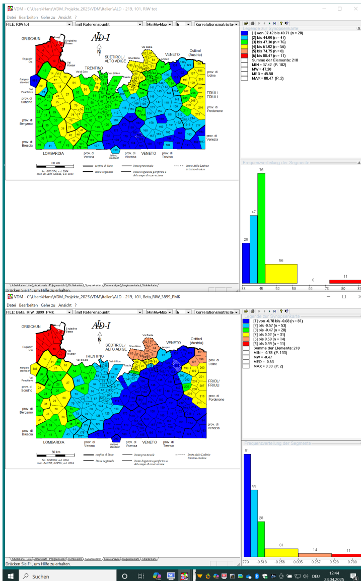
Karte 1 – Zwei Ähnlichkeitskarten zum ALD-I-Punkt 1 (Tschlin, Unterengadin) Oben (Alpha-Dialektometrie): Ähnlichkeitsmessung: RIW (Relativer Identitätswert) Unten (Beta-Dialektometrie): Ähnlichkeitsmessungen: RIW + PMK (Produkt-Moment-Korrelations-Koeffizient [nach Bravais-Pearson]) Visualisierung: Intervallalgorithmus MINWMAX 6-fach Korpus: 3.899 Arbeitskarten aus ALD-I (alle linguistischen Kategorien).
