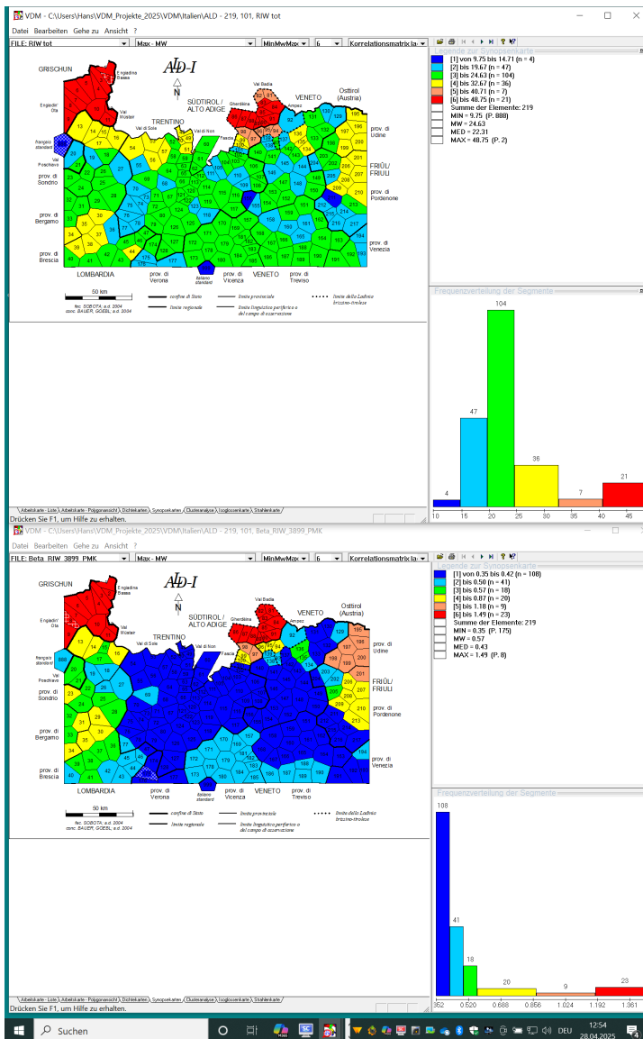
Karte 5 – Zwei Parameterkarten zum ALD-I: Synopse der Differenzen zwischen den Maxima (MAX) und den Mittelwerten (MW) der 219 Ähnlichkeitsverteilungen Oben (Alpha-Dialektometrie): Ähnlichkeitsmessung: RIW (Relativer Identitätswert) Unten (Beta-Dialektometrie): Ähnlichkeitsmessungen: RIW + PMK (Produkt-Moment-Korrelations-Koeffizient [nach Bravais-Pearson]) Visualisierung: Intervallalgorithmus MINMWMAX 6-fach Korpus: 3.899 Arbeitskarten aus ALD-I (alle linguistischen Kategorien).
