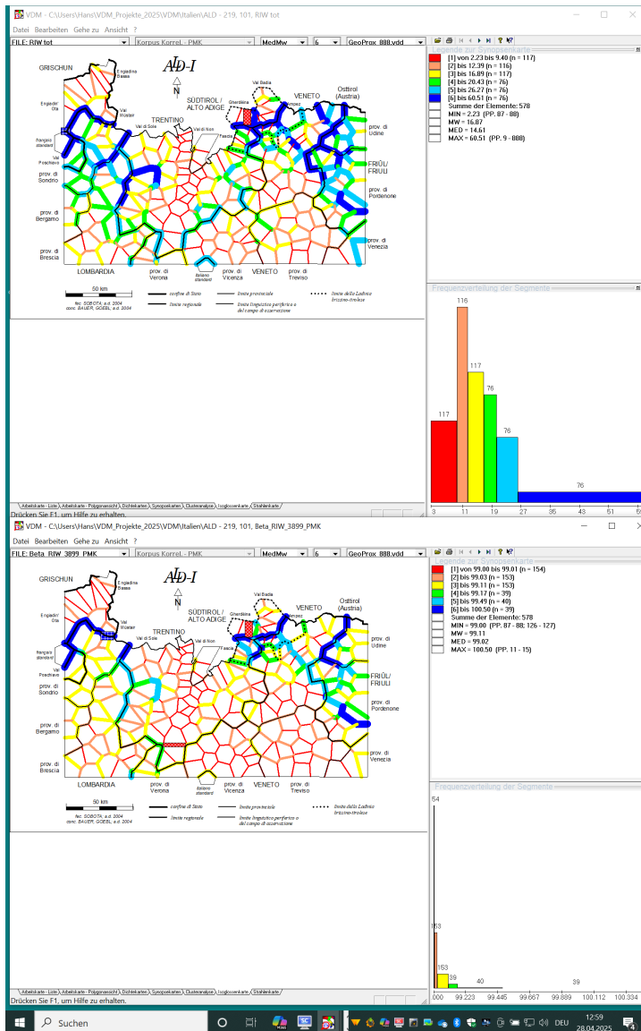
Karte 7 – Zwei Isoglossen-Synthesen zum ALD-I: Messung der interpunktuellen Distanzen Oben (Alpha-Dialektometrie): Distanzmessung: 1 - RIW (Relativer Identitätswert) Unten (Beta-Dialektometrie): Ähnlichkeitsmessungen: 1 - RIW + PMK (Produkt-Moment-Korrelations-Koeffizient [nach Bravais-Pearson]) Visualisierung: Intervallalgorithmus MEDMW 6-fach Korpus: 3.899 Arbeitskarten aus ALD-I (alle linguistischen Kategorien).
