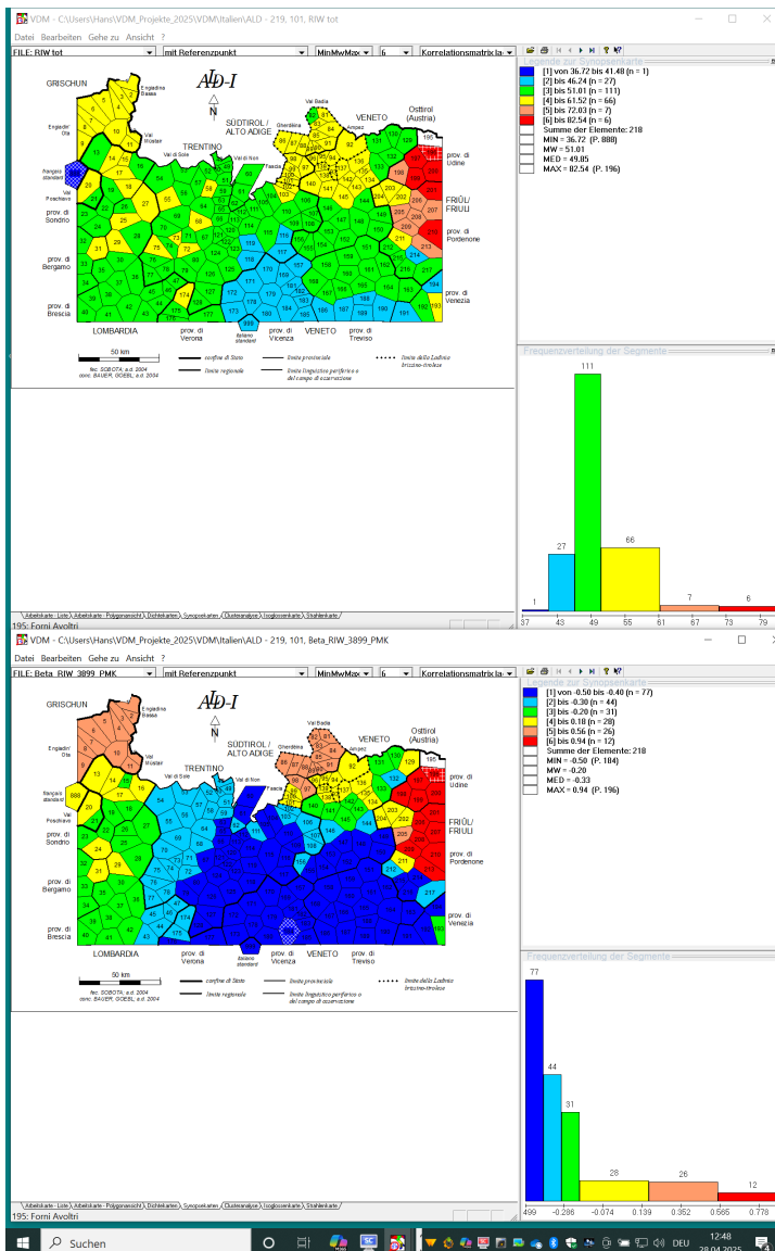
Karte 3 – Zwei Ähnlichkeitskarten zum ALD-I-Punkt 195 (Forni Avoltri, Friaul) Oben (Alpha-Dialektometrie): Ähnlichkeitsmessung: RIW (Relativer Identitätswert) Unten (Beta-Dialektometrie): Ähnlichkeitsmessungen: RIW + PMK (Produkt-Moment-Korrelations-Koeffizient [nach Bravais-Pearson]) Visualisierung: Intervallalgorithmus MINMWMAX 6-fach Korpus: 3.899 Arbeitskarten aus ALD-I (alle linguistischen Kategorien).
