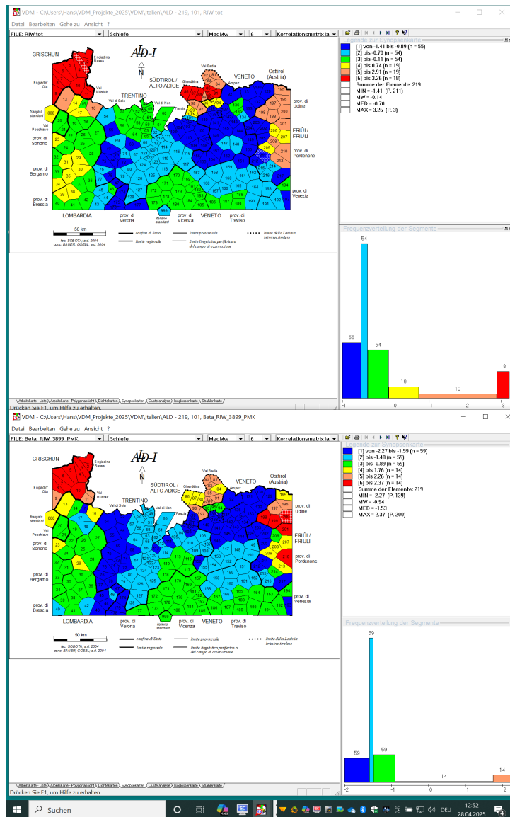
Karte 4 – Zwei Parameterkarten zum ALD-I: Synopse der Schiefen der 219 Ähnlichkeitsverteilungen Oben (Alpha-Dialektometrie): Ähnlichkeitsmessung: RIW (Relativer Identitätswert) Unten (Beta-Dialektometrie): Ähnlichkeitsmessungen: RIW + PMK (Produkt-Moment-Korrelations-Koeffizient [nach Bravais-Pearson]) Visualisierung: Intervallalgorithmus MEDMW 6-fach Korpus: 3.899 Arbeitskarten aus ALD-I (alle linguistischen Kategorien).
